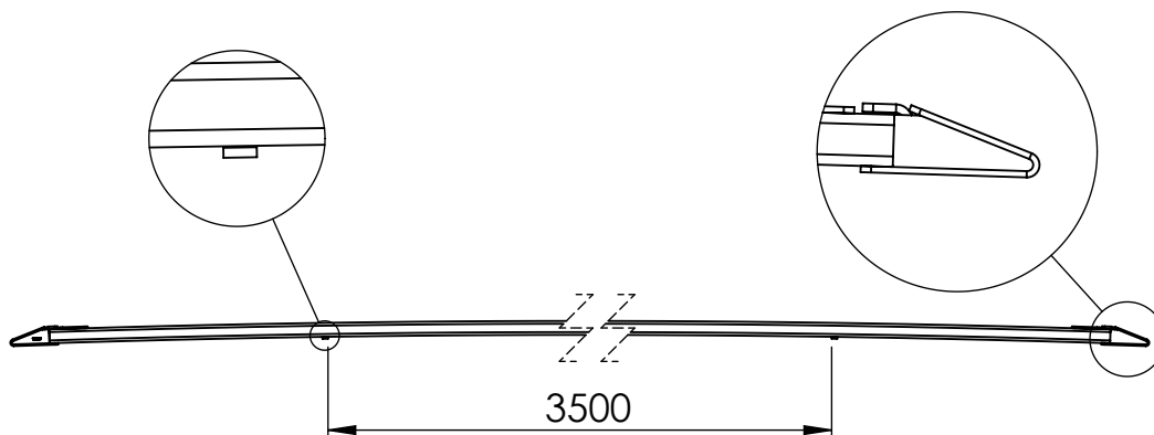
Påkörningsramp 20°
