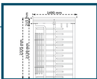
Ritning med mål. Passagehöjd är 2m. Passagebredden 0,6m.
